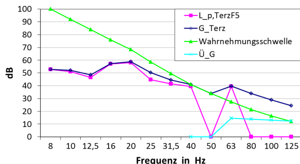
Abbildung 3: Auswertung nach E DIN 45680 [2] mit den gemessenen Terzpegeln L_{p,\text{TerzF5}} der Wahrnehmungsschwelle, dem terzabhängigen Wert des Lautheitsspektrums G_{\text{Terz}} und der gewichteten Schwellenüberschreitung \ddot{U}_G .
