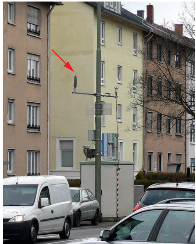
Abbildung 5.2-1: Messstation der LUBW zur Erfassung von Straßenverkehrslärm in Karlsruhe, Reinhold-Frank-Straße. Der Pfeil zeigt die Lage des Mikrofons, im Hintergrund Wohnbebauung. Foto: LUBW
