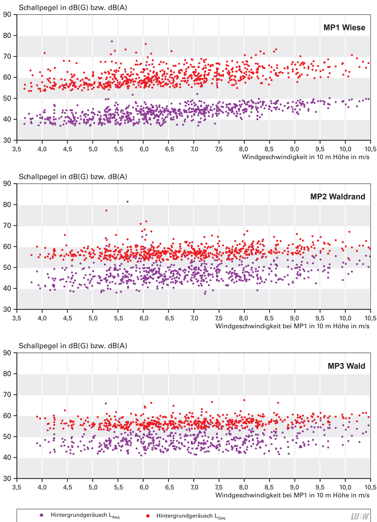
Abbildung 8.1-7: Hörschallpegel (A-Pegel) und Infraschallpegel (G-Pegel) in Abhängigkeit von der Windgeschwindigkeit für die drei Messpunkte MP1 (Wiese), MP2 (Waldrand) und MP3 (Wald). Dargestellt sind die G-Pegel (rote Punkte) und die A-Pegel (violette Punkte). Die Windmessung erfolgte stets am Messpunkt MP1 (Wiese).
