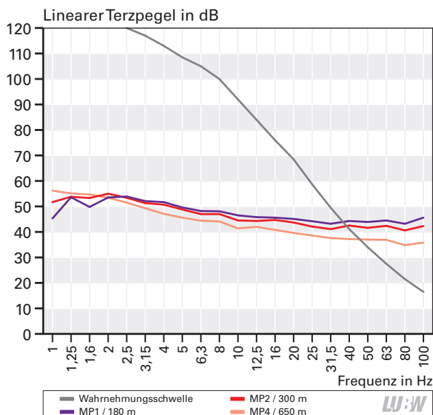
Abbildung 4.5-11: Terzspektren des Gesamtgeräusches an den Messpunkten MP1 (180 m), MP2 (300 m) und MP4 (650 m) der WEA 4, Wahrnehmungsschwelle nach Tabelle A3-1 zum Vergleich. Die Messwerte wurden gemäß Abschnitt 4.1 korrigiert.
