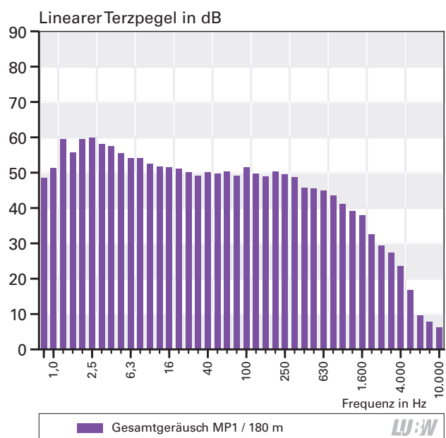
Abbildung 4.5-10: Terzspektr von Gesamtgeräusch und Hintergrundgeräusch im Nahbereich der Windenergieanlage WEA 4
