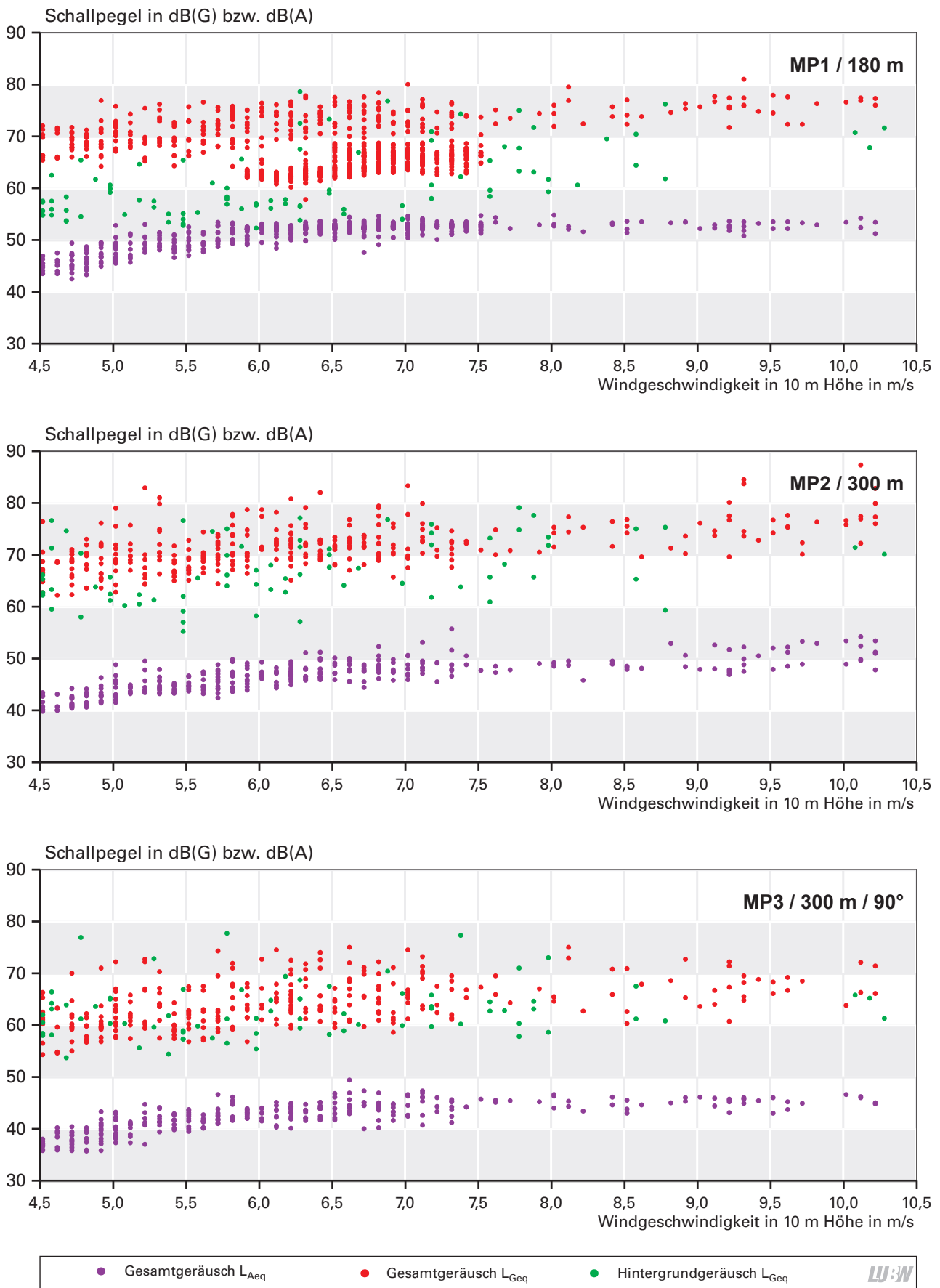
Abbildung 4.4-6: Hörschallpegel (A-Pegel) und Infraschallpegel (G-Pegel) in Abhängigkeit von der Windgeschwindigkeit für die Windenergieanlage WEA 3. Dargestellt sind die G-Pegel bei eingeschalteter Anlage (rote Punkte) und bei ausgeschalteter Anlage (grüne Punkte) sowie die A-Pegel bei eingeschalteter Anlage (violette Punkte).
