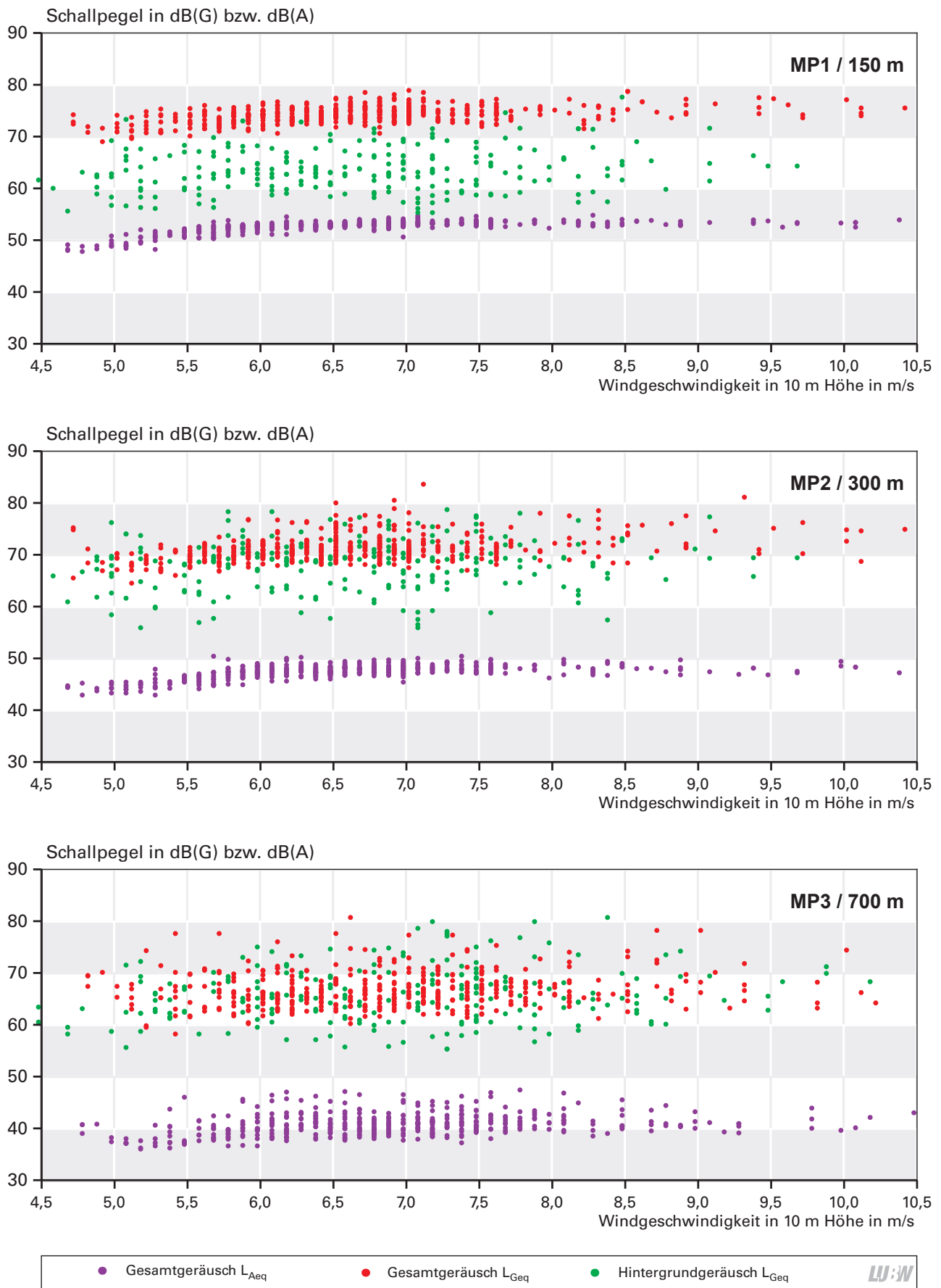
Abbildung 4.2-6: Hörschallpegel (A-Pegel) und Infraschallpegel (G-Pegel) in Abhängigkeit von der Windgeschwindigkeit für die Windenergieanlage WEA 1. Dargestellt sind die G-Pegel bei eingeschalteter Anlage (rote Punkte) und bei ausgeschalteter Anlage (grüne Punkte) sowie die A-Pegel bei eingeschalteter Anlage (violette Punkte).
