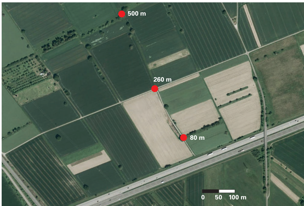
Abbildung 5.3-1: Lage der Messpunkte an der Bundesautobahn A5 südlich von Karlsruhe bei Malsch, mit Angabe der Abstände der Mikrofonpositionen zur Autobahnmitte. Die Gemeinde Malsch befindet sich außerhalb des Bildes links unten. Oberhalb des Bildausschnittes verläuft die Bundesstraße B3. Bildquelle: LUBW, LGL
