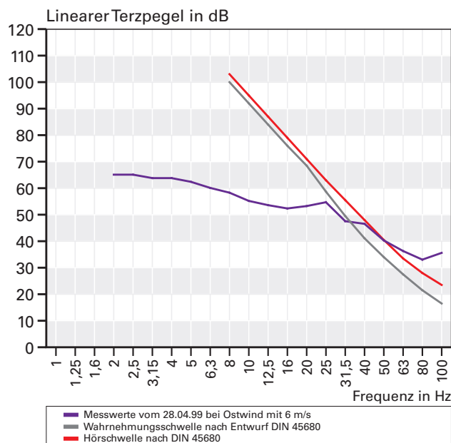
Abbildung 4.9-3: Das untersuchte Windrad erzeugt Schallwellen, die von auf einem Balkon in 250 m Entfernung stehenden Menschen nur oberhalb 40 Hz gehört werden können. Der Infraschallbereich ist hier nicht wahrnehmbar, da er deutlich unterhalb der Wahrnehmungsschwelle liegt. Quelle: [15]
