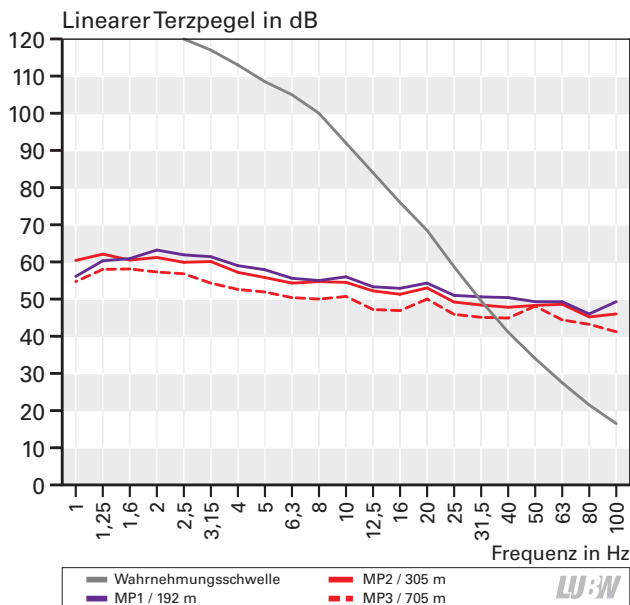
Abbildung 4.7-5: Terzspektrn des Gesamtgeräuschs an den Messpunkten MP1 (192 m), MP2 (305 m) und MP3 (705 m) der WEA 6, Wahrnehmungsschwelle nach Tabelle A3-1 zum Vergleich. Die Messwerte wurden gemäß Abschnitt 4.1 korrigiert.
