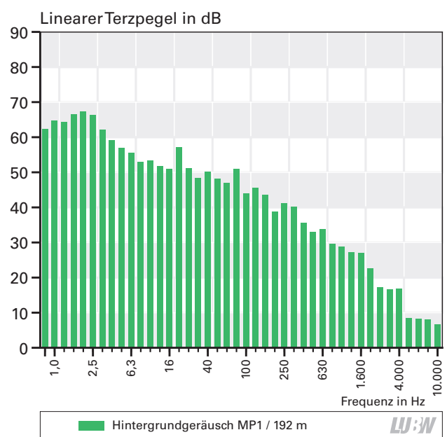
Abbildung 4.7-4: Terzspektr von Gesamtgeräusch und Hintergrundgeräusch im Nahbereich der Windenergieanlage WEA 6
