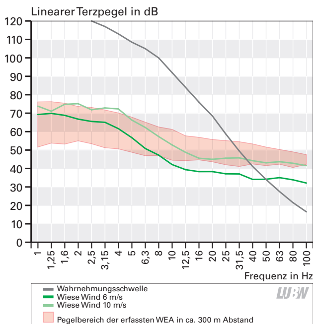
Abbildung 2-5: Vergleich der Geräuschesituation im freien Feld (ohne Quellenbezug) mit dem Pegelbereich von WEA in etwa 300 m Abstand sowie der Wahrnehmungsschwelle nach Tabelle A3-1 hinsichtlich Infraschall und tieffrequenten Geräuschen. Zu Messkorrekturen bei WEA siehe Abschnitt 4.1.
