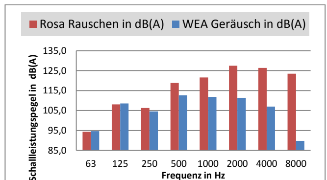
Abbildung 1: Oktavbänder des Lautsprechers mit rosa Rauschen (Rot) und WEA Geräusch (Blau) normiert auf den Schallleistungspegel in dB(A).
